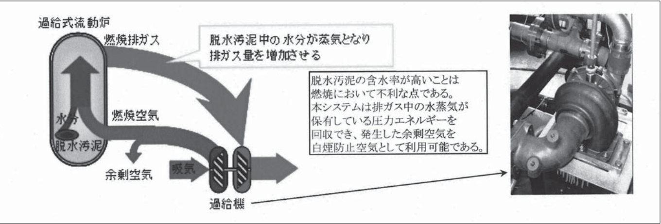
図3 過給機によるエネルギー回収 Fig.3 Energy recovery by the turbocharger
