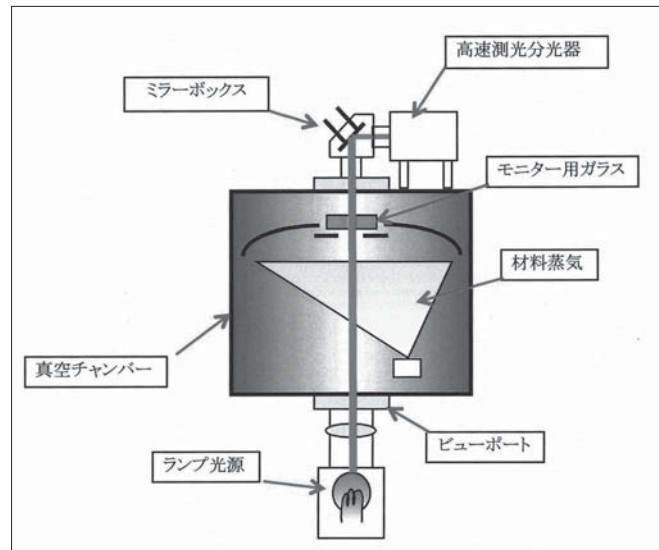
図10 真空中での光学式膜厚モニターの模式図 Fig.10 Schematic drawing of optical monitor system in vacuum
