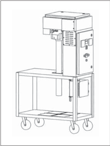
図3 コリメートビーム照射ユニット Fig.3 Collimated Beam Unit
