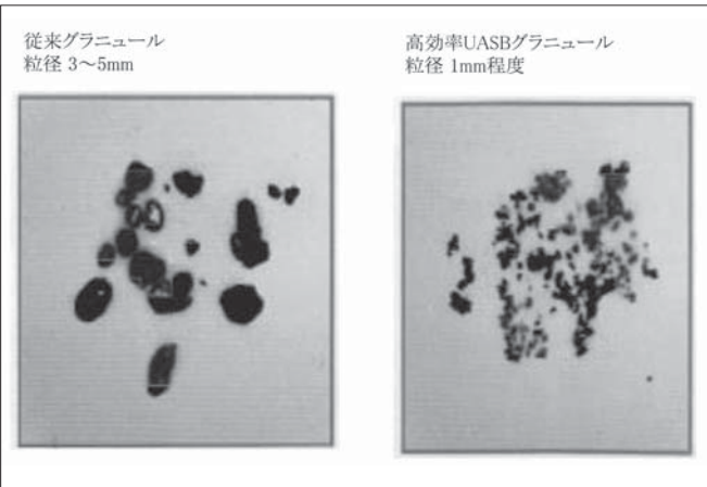
図2 グラニュール写真 Fig.2 Photo of granules.
