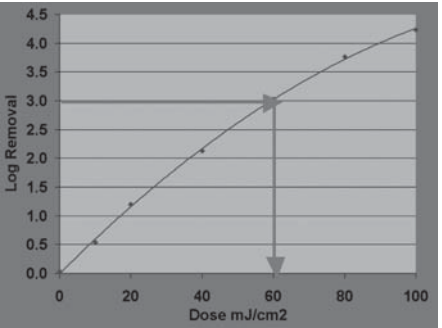
図4 紫外線照射量 vs MS2 不活化率グラフ Fig.4 UV dose vs Log Removal of MS2
