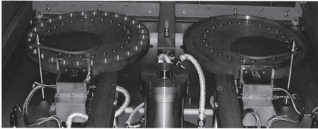
図7 電子ビームガン、ルツボの配置(中央：プラズマガン、左右：ルツボ) Fig.7 Arrangement of electron beam gun and melting pot (Center:plasma source, Both side of gun:Melting pot)
