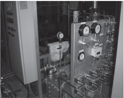
図9 過給機ユニット外観 Fig.9 Photo of turbocharger unit
