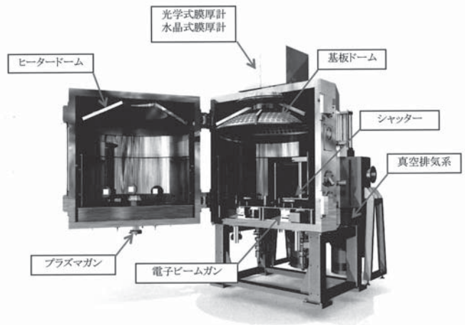
図6 XLS1500PAの内部イメージ Fig.6 Internal view of XLS1500PA
