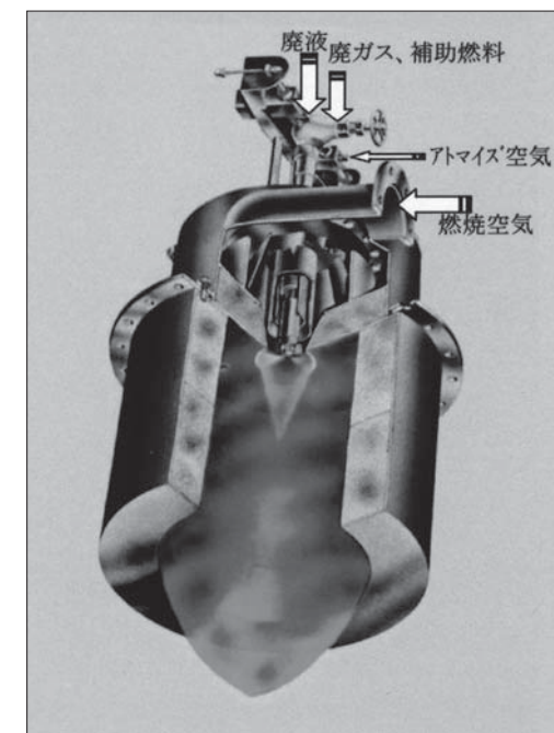
図3 ボルテックスバーナー説明図 Fig.3 Explanatory drawing of Vortex Burner
