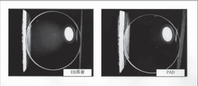
図17 外観品質(散乱状態)の比較 Fig.17 Comparison of light scattering
