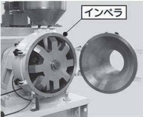
図4 サイクロンミル 分解時の様子 Fig.4 Cyclone mill state during disassembly
