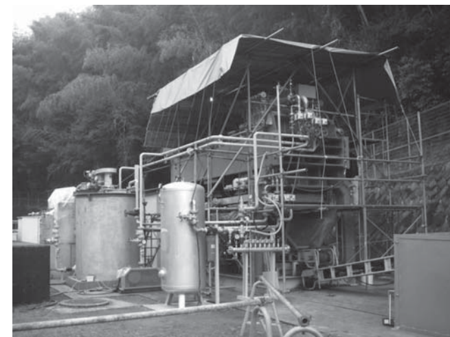
図3 実験プラント写真 Fig.3 Photo of Experiment plant
