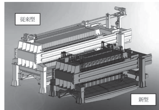
図4 従来型と新型DCフィルタの全体イメージ Fig.4 Comparison of New and Conventional DC filter
