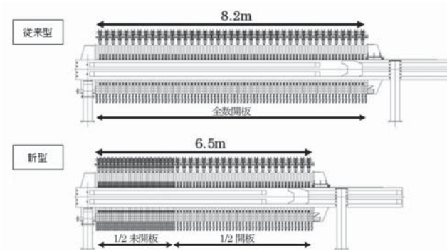
図2 2段階排出による省スペース効果(ろ過面積400m 2 ) Fig.2 Space-saving Effect of Two-stage Discharge(filtration area 400m 2 )
