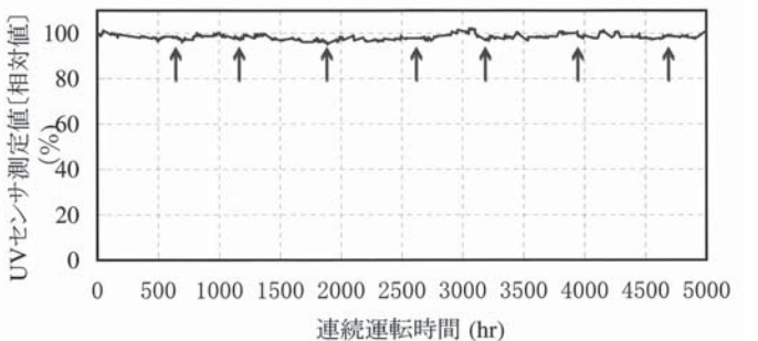
図10 UV センサ測定値の経時変化 Fig.10 UV intensity data of duty sensor
