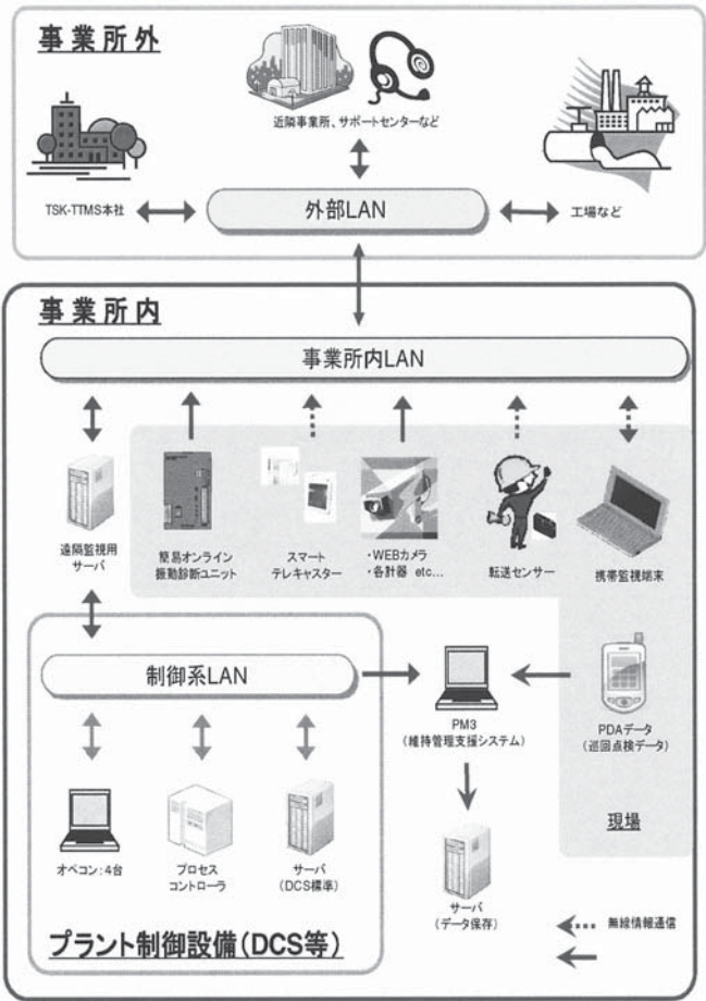
図17 現場システム全体概要図 Fig.17 Outline of the whole system for site
