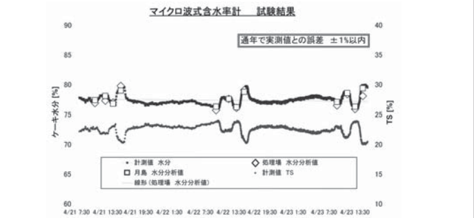
図13 水分計の実測データ Fig.13 Monitoring data of water content meter
