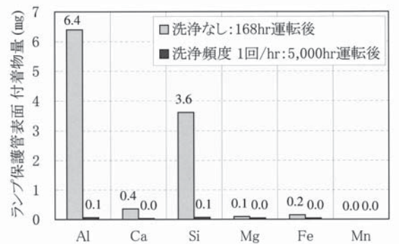
図12 ランプ保護管付着成分 分析結果 Fig.12 Attached metals amount on the lamp sleeve
