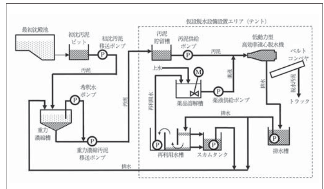
図4 仮設脱水設備 概略フロー Fig.4 Overview flow of the temporary dewatering plant
