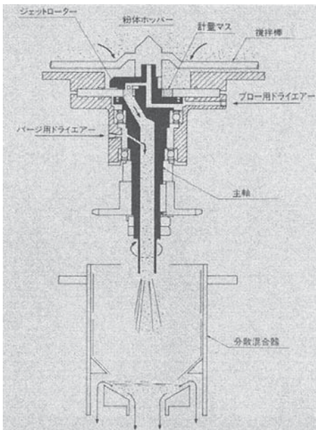
図13 粉末系高分子凝集剤の溶解作業に用いられる定量供給機及び分散混合器 6)
