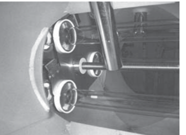
図5 紫外線消毒装置 センチネル300型 照射槽内部 Fig.5 Internal design of UV disinfection system SENTINEL 12
