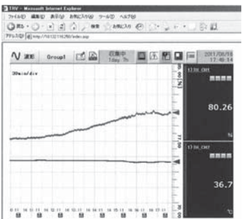
図15 ケーキ水分のモニタリング画面 Fig.15 Monitoring of water content meter
