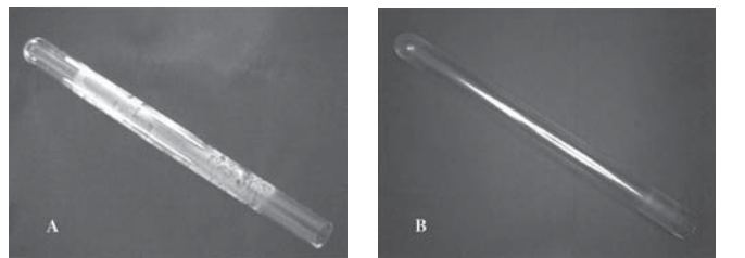
図11 ランプ保護管写真 A) 洗浄なし-168hr 運転後、 B) 洗浄あり【1回/hr】-5,000hr 運転後 Fig.11 Lamp sleeve: A) No cleaning (after 168hr), B) Hourly cleaning (after 5,000hr)
