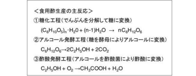
図1 食酢生産の主反応
