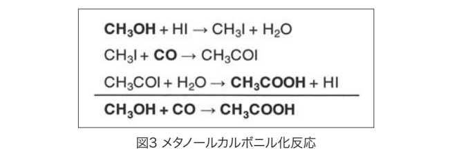
図3 メタノールカルボニル化反応
