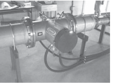
図4 紫外線消毒装置 センチネル300型 照射槽外観 Fig.4 Exterior design of UV disinfection system SENTINEL 12
