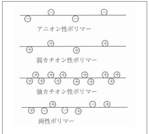
図11 ポリマー凝集剤の分子構造のイメージ Fig.11 Image of molecular structure of polymer flocculant
