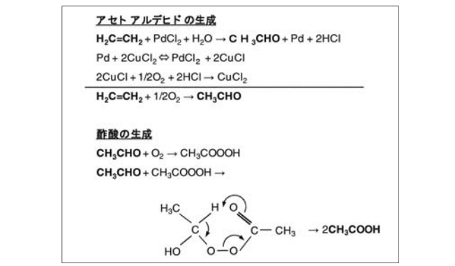
図2 アセトアルデヒド酸化法の反応
